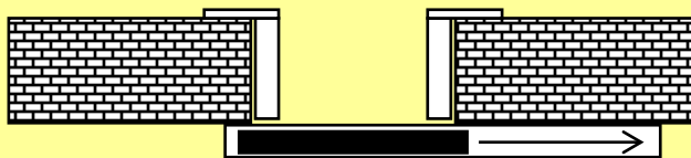
1-НО СТВОРЧАТАЯ ДВЕРЬ - СДВИЖЕНИЕ ВДОЛЬ СТЕНЫ С ОБРАМЛЕНИЕМ ПРОЁМА
