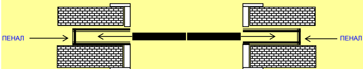
2-У СТВОРЧАТАЯ ДВЕРЬ - СДВИЖЕНИЕ В МЕТАЛЛ. ПЕНАЛЫ С ОБРАМЛЕНИЕМ ПРОЁМА С 2-УХ СТОРОН ПРОЁМА
