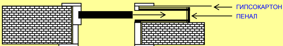
1-НО СТВОРЧАТАЯ ДВЕРЬ - СДВИЖЕНИЕ В МЕТАЛЛИЧЕСКИЙ ПЕНАЛ С ОБРАМЛЕНИЕМ ПРОЁМА С 1-ОЙ СТОРОНЫ
