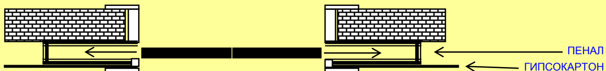
2-У СТВОРЧАТАЯ ДВЕРЬ - СДВИЖЕНИЕ В МЕТАЛЛ. ПЕНАЛЫ С ОБРАМЛЕНИЕМ ПРОЁМА С 1-ОЙ СТОРОНЫ ПРОЁМА
